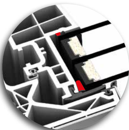
I-tec Vitrage
