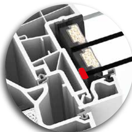
I-tec Vitrage
