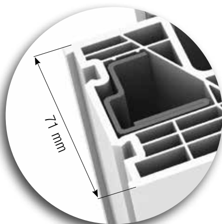
Epaisseur dormant
