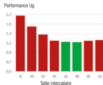
Intercalaire ISO
